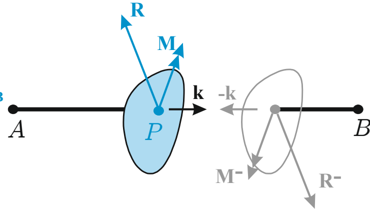
Forze interne
